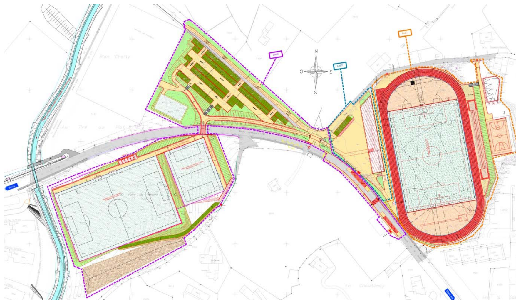
Plan général du site
